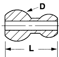
TYP 2 passar Snap-Loc 1/4"
