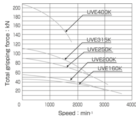
Spännkraftsdiagram
