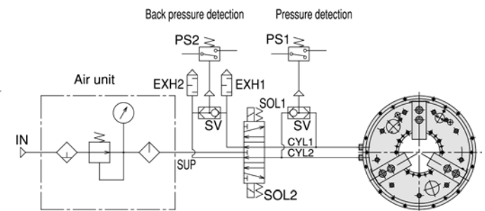
Rekommenderat kopplingsschema ( Pneumatik )
