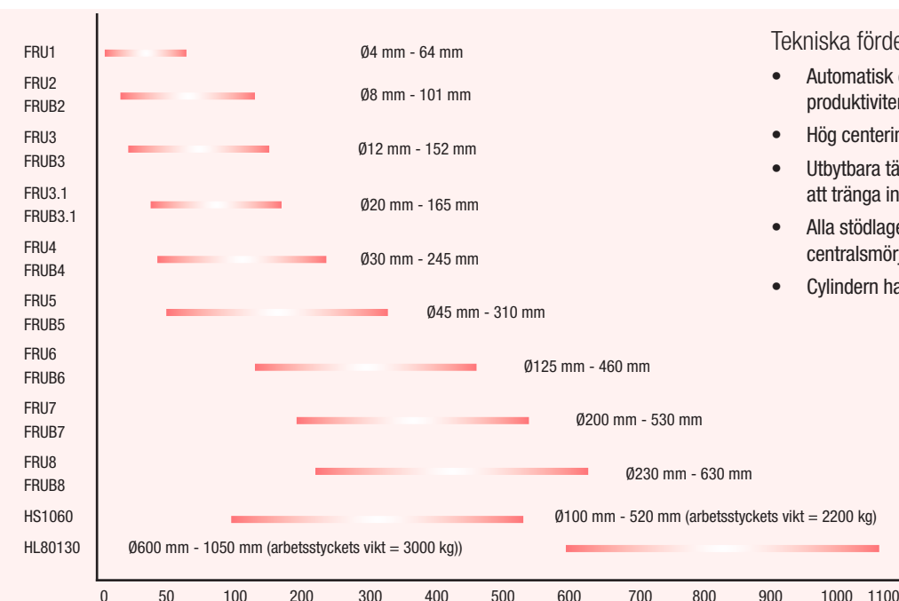
Arbetsområden (mm)
